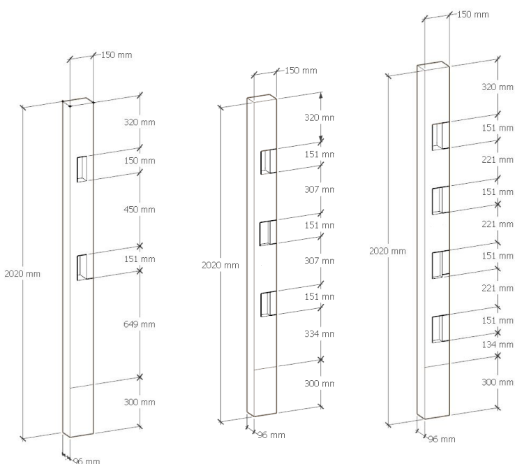
MEDIDAS POSTE
